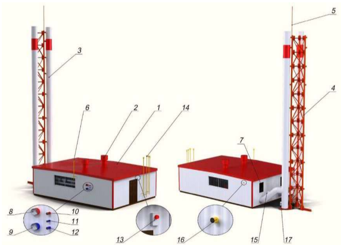
Рис. 1. Внешний вид блочно-модульной котельной в базовом исполнении
